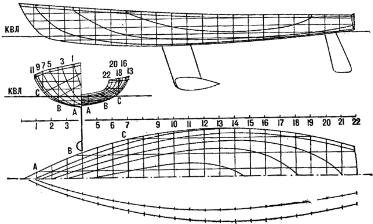
Рис. 85. Теоретический чертеж килевой яхты класса «Темпест»
