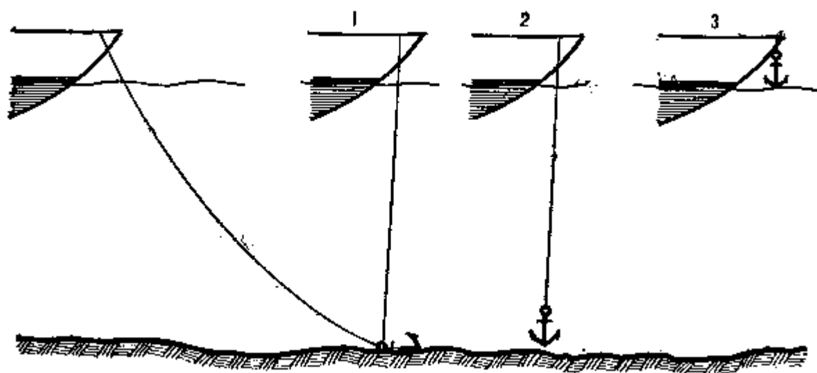
Рис. 127, Схема съёмки с якоря:
