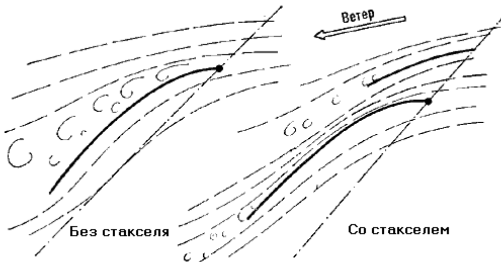
Рис. 97. Работа стакселя
