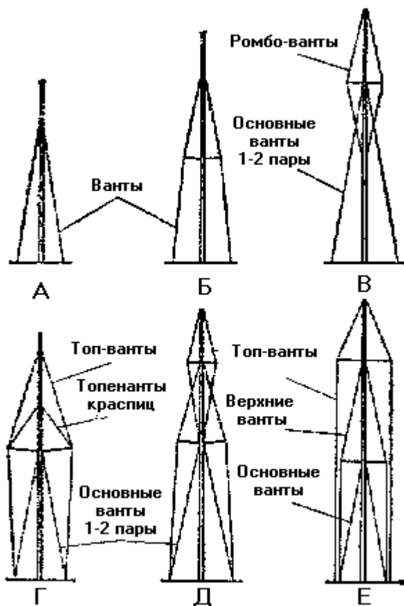
Рис. 38. Проводка вант:
