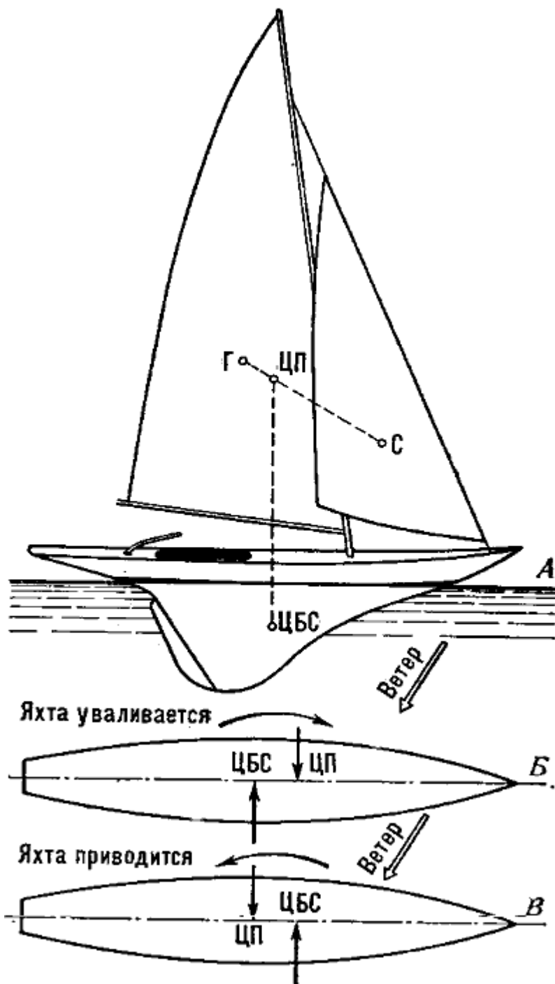
Рис. 99. Центровка яхты
