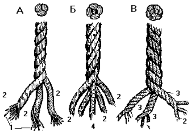
Рис. 55. Растительные тросы:
