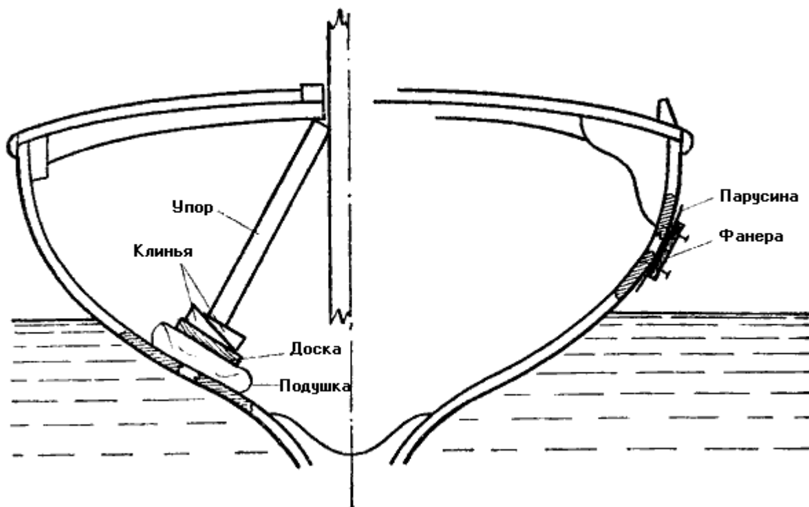
Рис. 136. Заделка надводной и подводной пробоины
