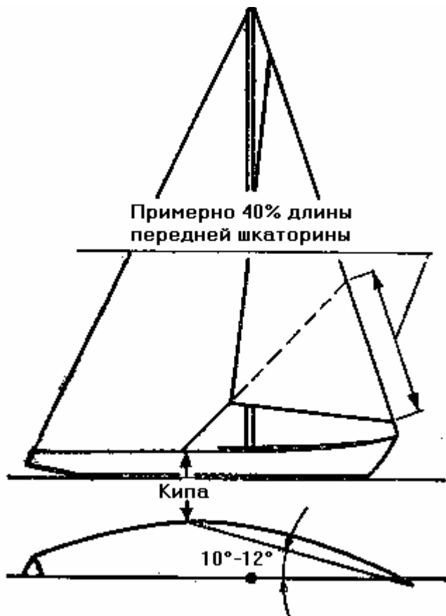
Рис. 46. Проводка стаксель-шкотов
