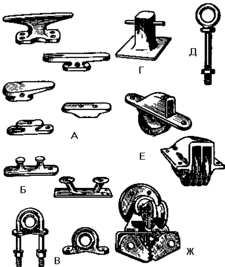
Рис. 50. Дельные вещи:
