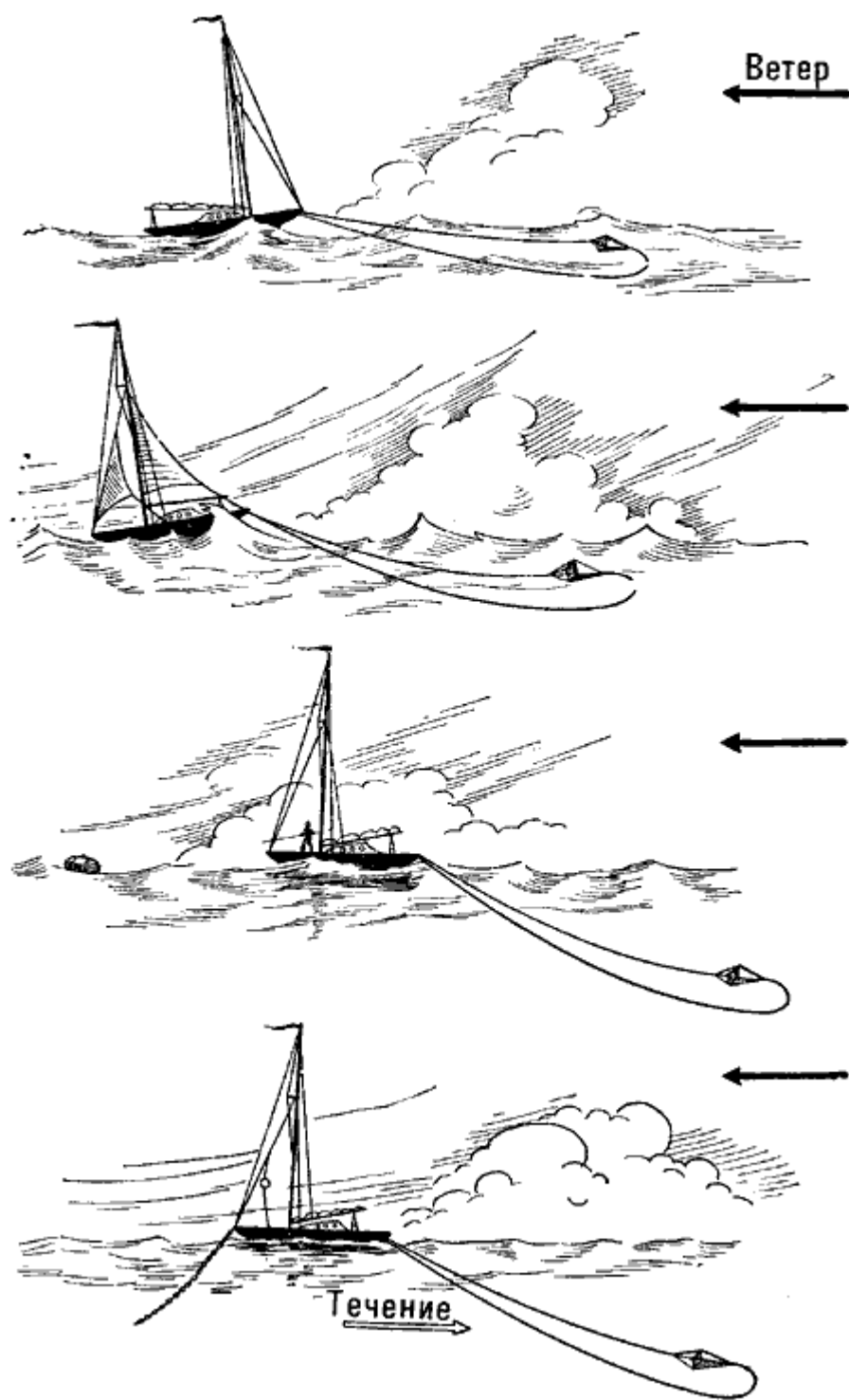
Рис. 118. Некоторые случаи применения плавучего якоря
