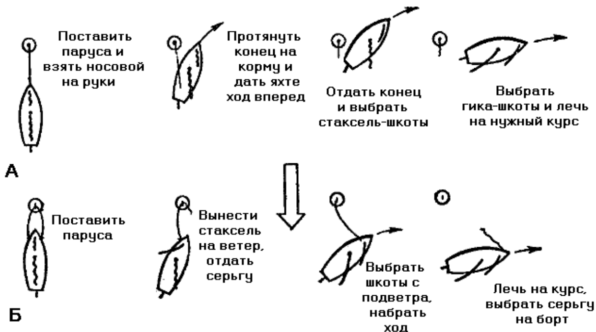
Рис. 122. Отход от буя или бочки А. — если яхта стояла на носовом, закрепленном на бочке, конце; Б — если яхта стояла на носовом конце, заложенном серьгой
