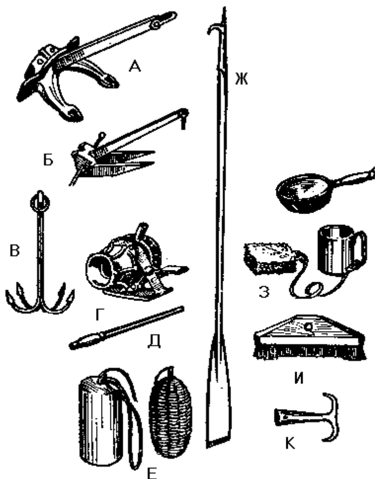
Рис. 54. Некоторые предметы снабжения и оборудования яхты: А, Б — якоря без штоков; В — кошка; Г — брашпиль; Д — вымбовка; Е—кранцы; Ж—весло с отпорным крюком; З — черпаки-лейки; И — щетка для мытья палубы; К — отпорный крюк
