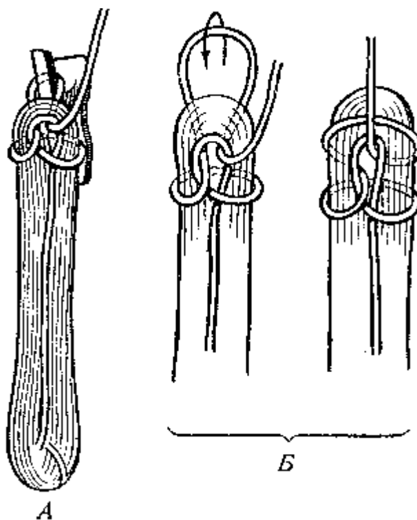
Рис. 103. Фал в походной бухте
