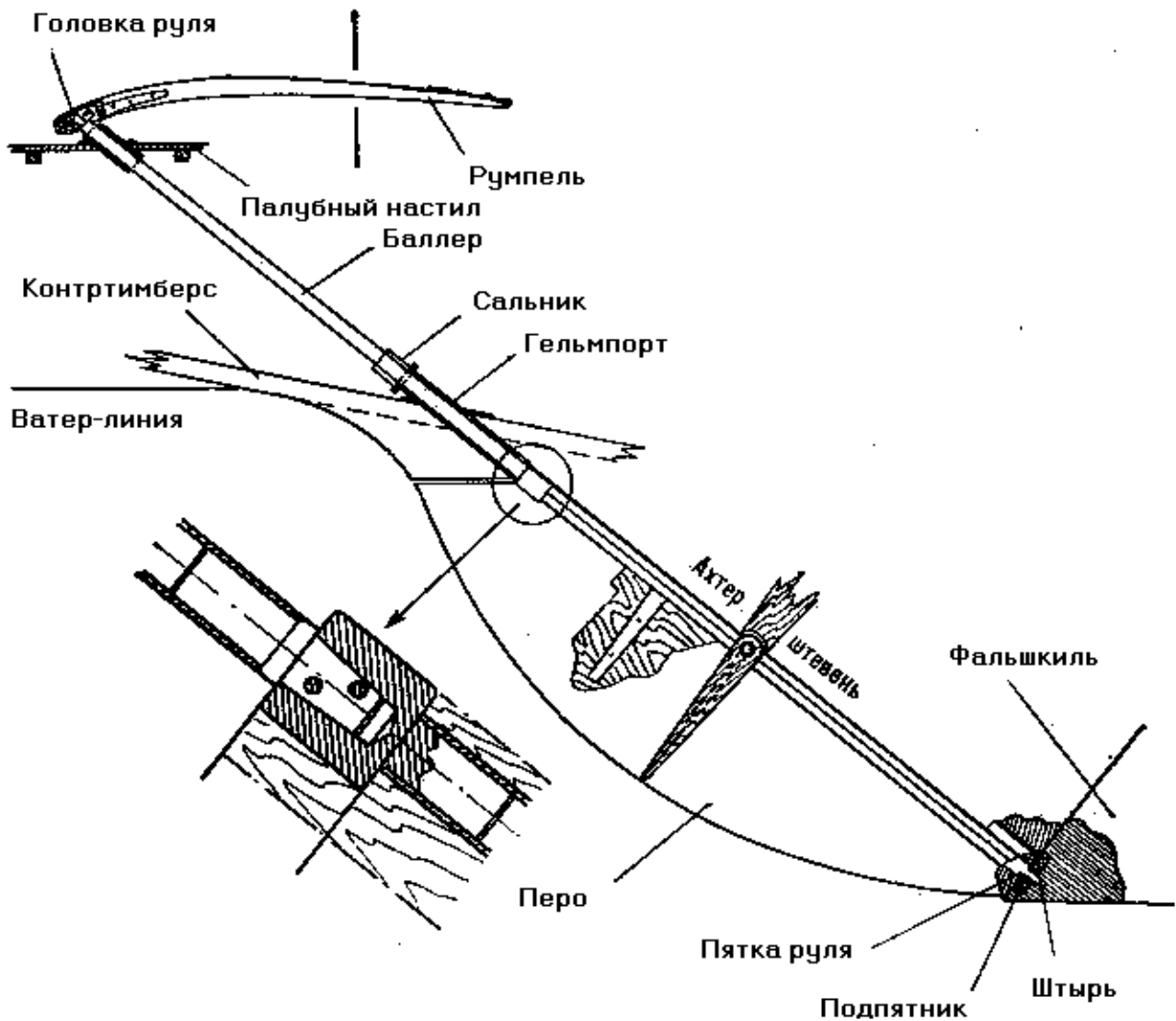
Рис. 31. Руль килевой яхты и его части
