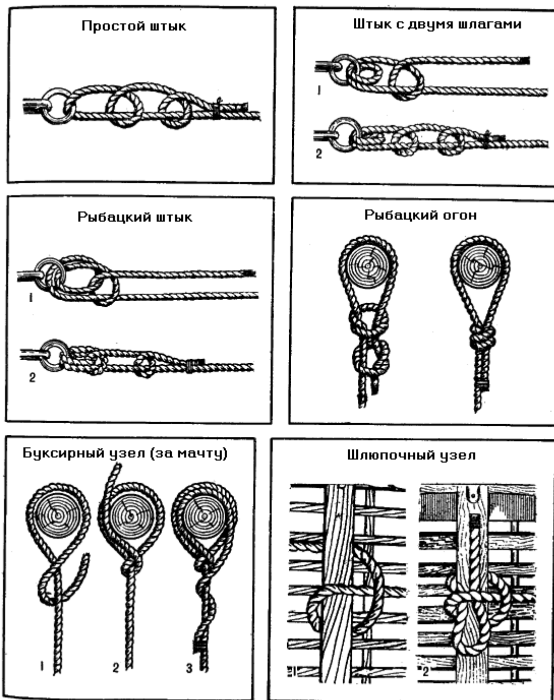
Рис. 60. Узлы для швартовки в буксировки
