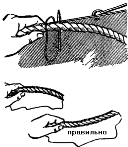
Пришивание лик-троса
