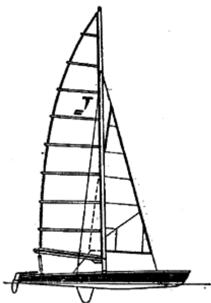
Рис. 16. Катамаран-моготип “Торнадо”
