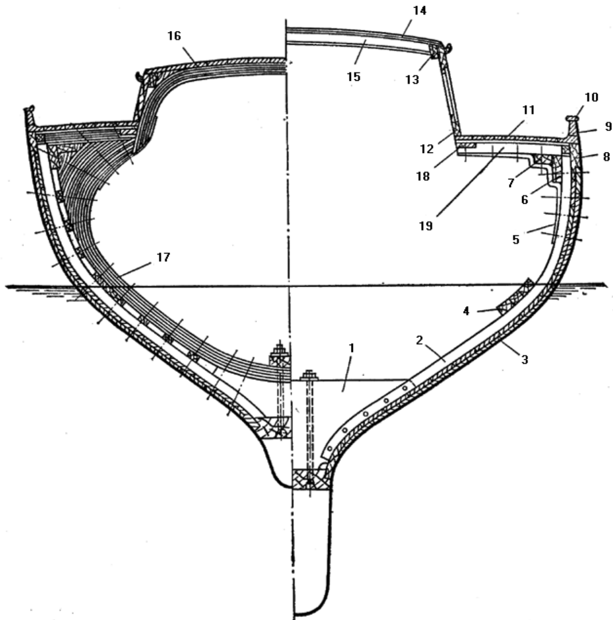
Рис. 27. Поперечный разрез деревянной кругло-шпангоутной яхты:
