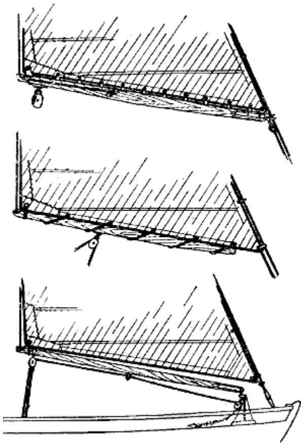
Рис. 43. Рейки стакселей
