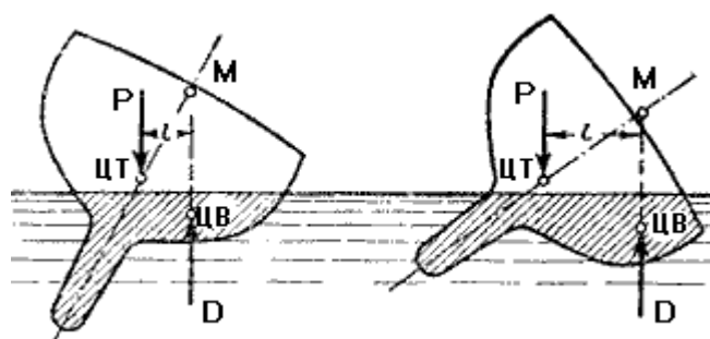
Рис. 80. Остойчивость килевой яхты
