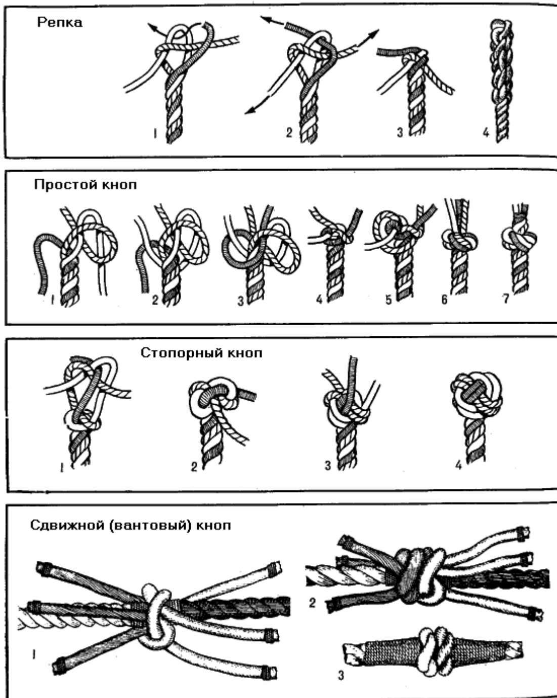
Рис. 69, Кнопы
