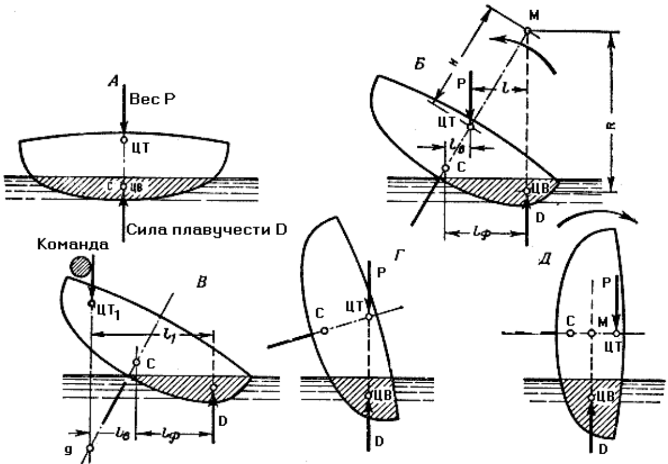
Рис. 78. Остойчивость швертбота
