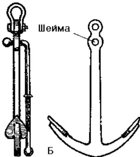
Рис 52. Адмиралтейский якорь и его части А - в рабочем положении Б - в походном положении
