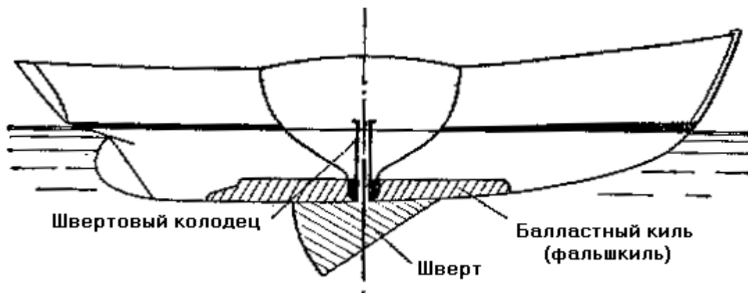
рис. 6. Яхта-компромисс
