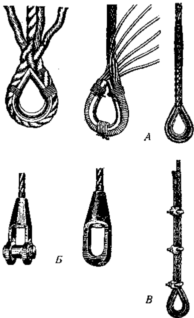
Рис. 68. Заделка концов такелажа: А — введение коуша, Б — концевые обоймы, В — сжимы для стальных тросов
