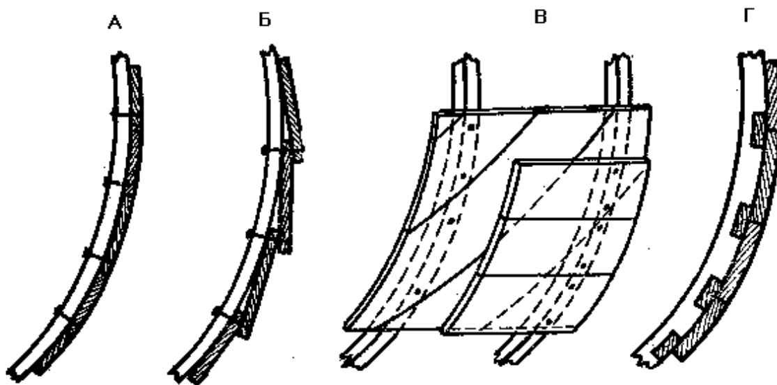
Рис. 29. Виды обшивки:
