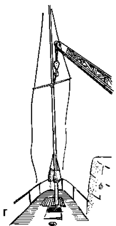
ис. 75. Способы подъема и спуска яхты: А — на слипе; Б — краном с внутренним стропом; В — краном наружным стропом; Г — постановка мачты краном.
