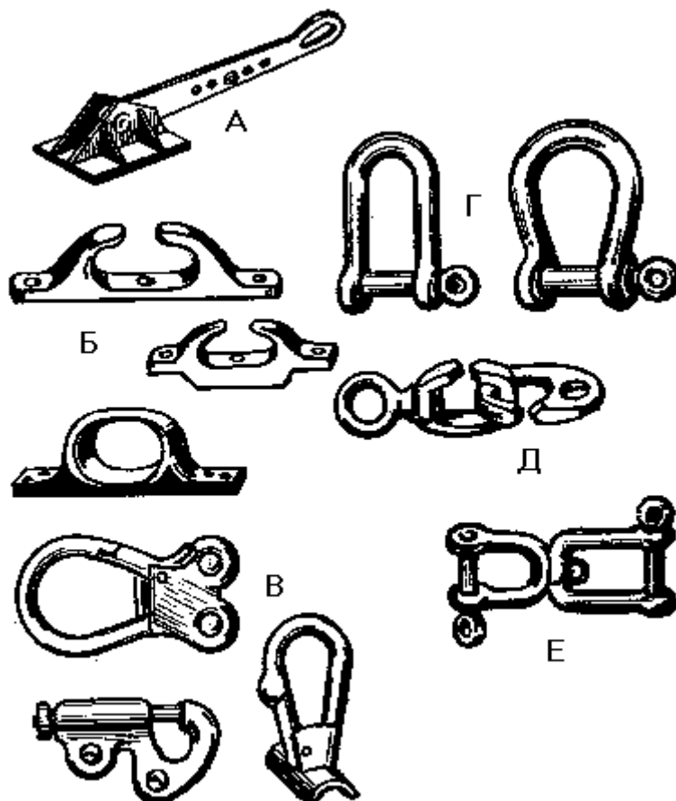
Рис. 51. Дельные вещи:
