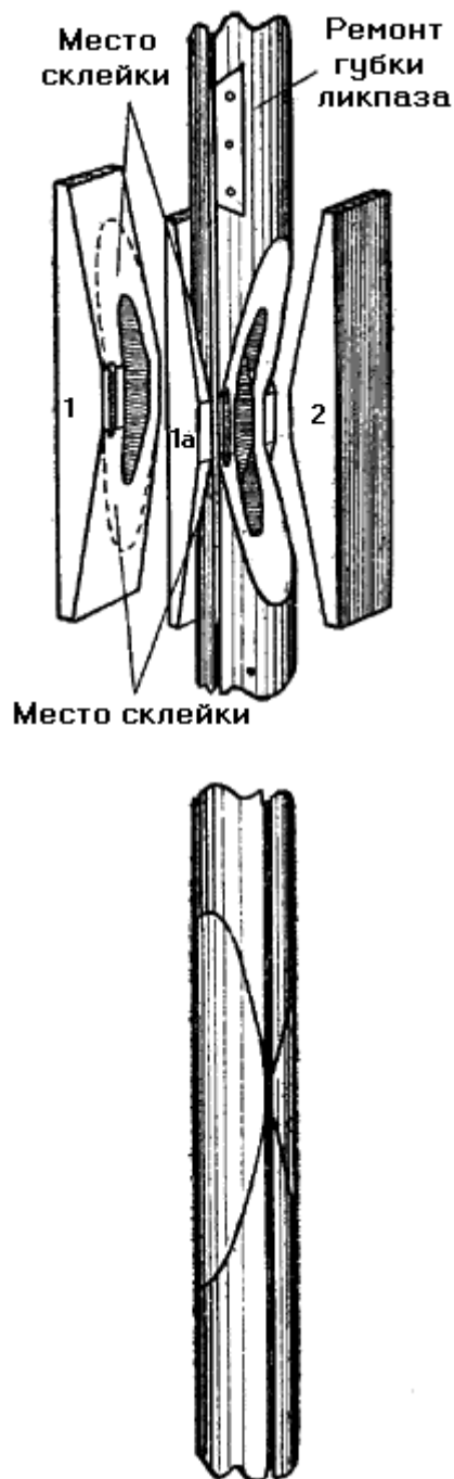
Рис. 74. Склеивание сломанной мачты
