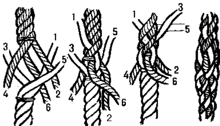
Рис. 63. Короткий спlesenь на растительном тросе
