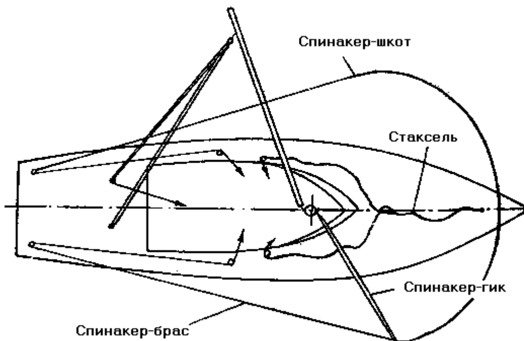
Рис. 48. Такелаж спинакер-гика
