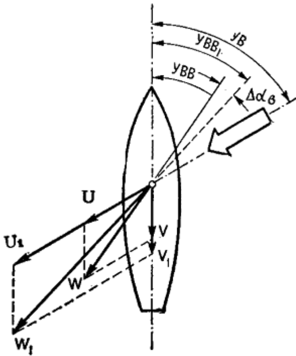
Рис. 91. При слабом ветре вымпел отклоняется больше, чем при сильном
