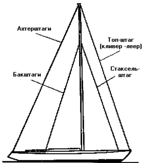
Рис. 39. Проводка штагов
