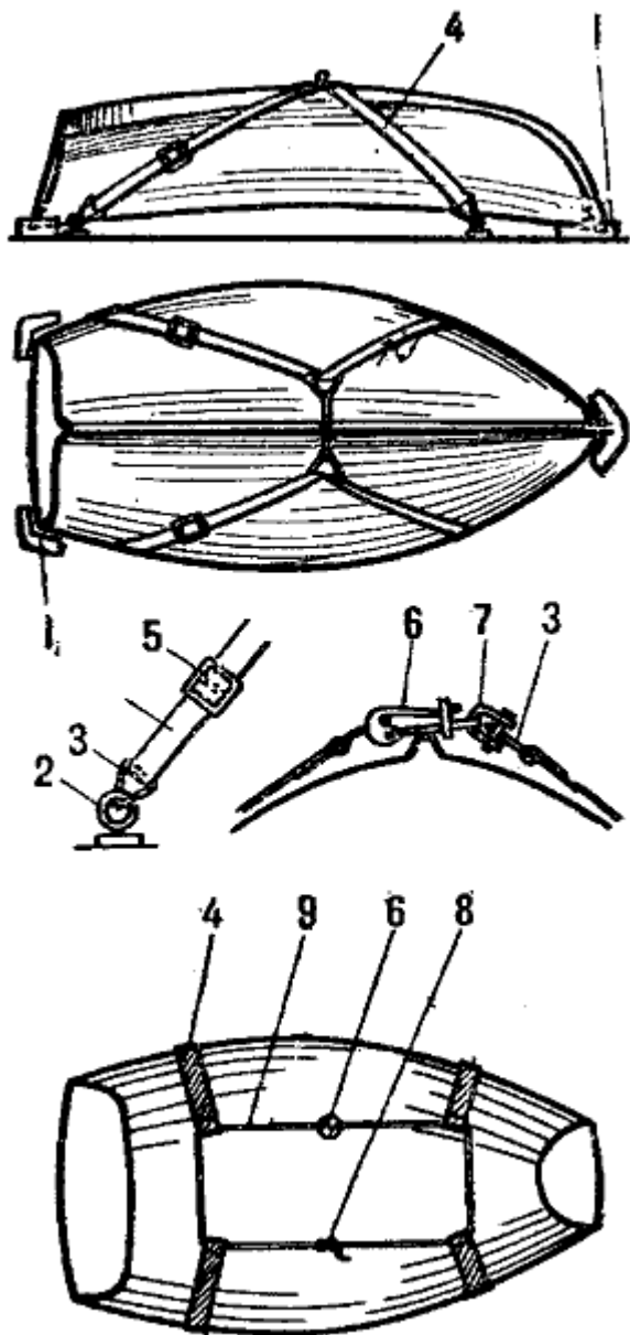
Рис. 132. Два способа крепления тузика по-походному: 1 — подушки; 2 — обушок, 3 — треугольное звено; 4 — парусиновый ремень (найтов); 5 — натяжная пряжка; 6 — быстроотдающей глаголь-гак; 7 — такелажная скоба; 8 — рифовый узел; 9 — растительный или синтетический лить
