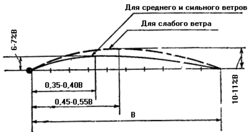
Рис. 96. Профиль паруса
