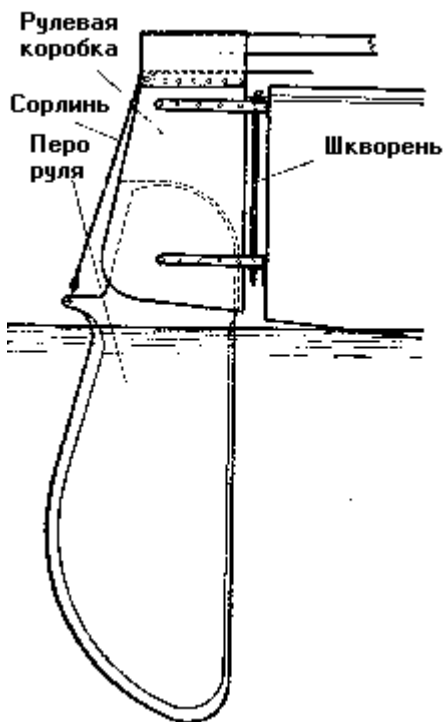
Рис. 32. Устройство подвесного руля швурбота
