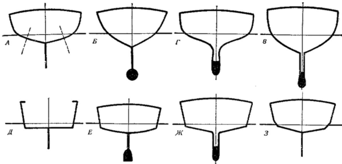
Рис. 9. Формы мидель-шпангоутов.
