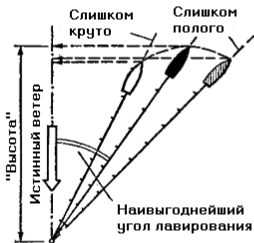
Рис. 106. Наивыгоднейший курс при лавировке. Несмотря на то что белая яхта идет круче, а полосатая быстрее, черная имеет наибольшую скорость лавировки
