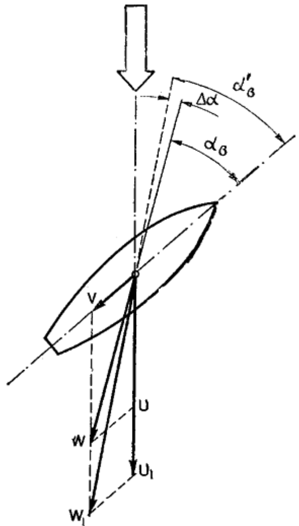
Рис. 92. В полосе сильного ветра можно идти круче
