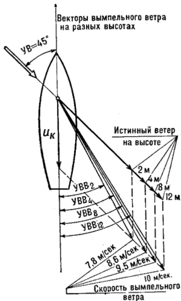
Рис. 93. Изменение вымпельного ветра с высотой
