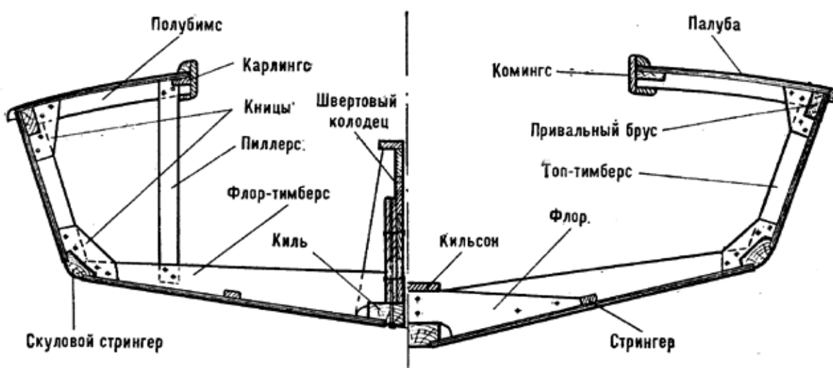
Рис. 28 Поперечный разрез швертбота-шарпи с фанерной обшивкой
