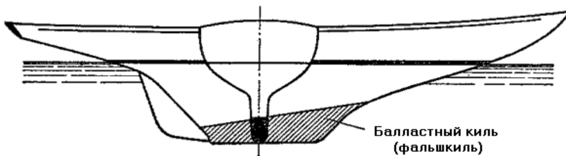
Рис. 4. Килевая яхта
